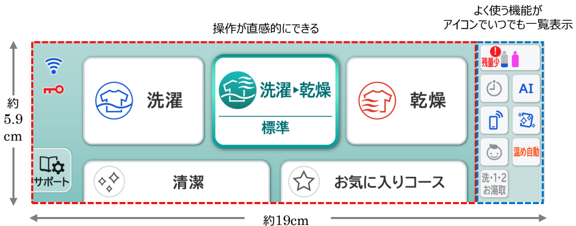
図1：ホーム画面
