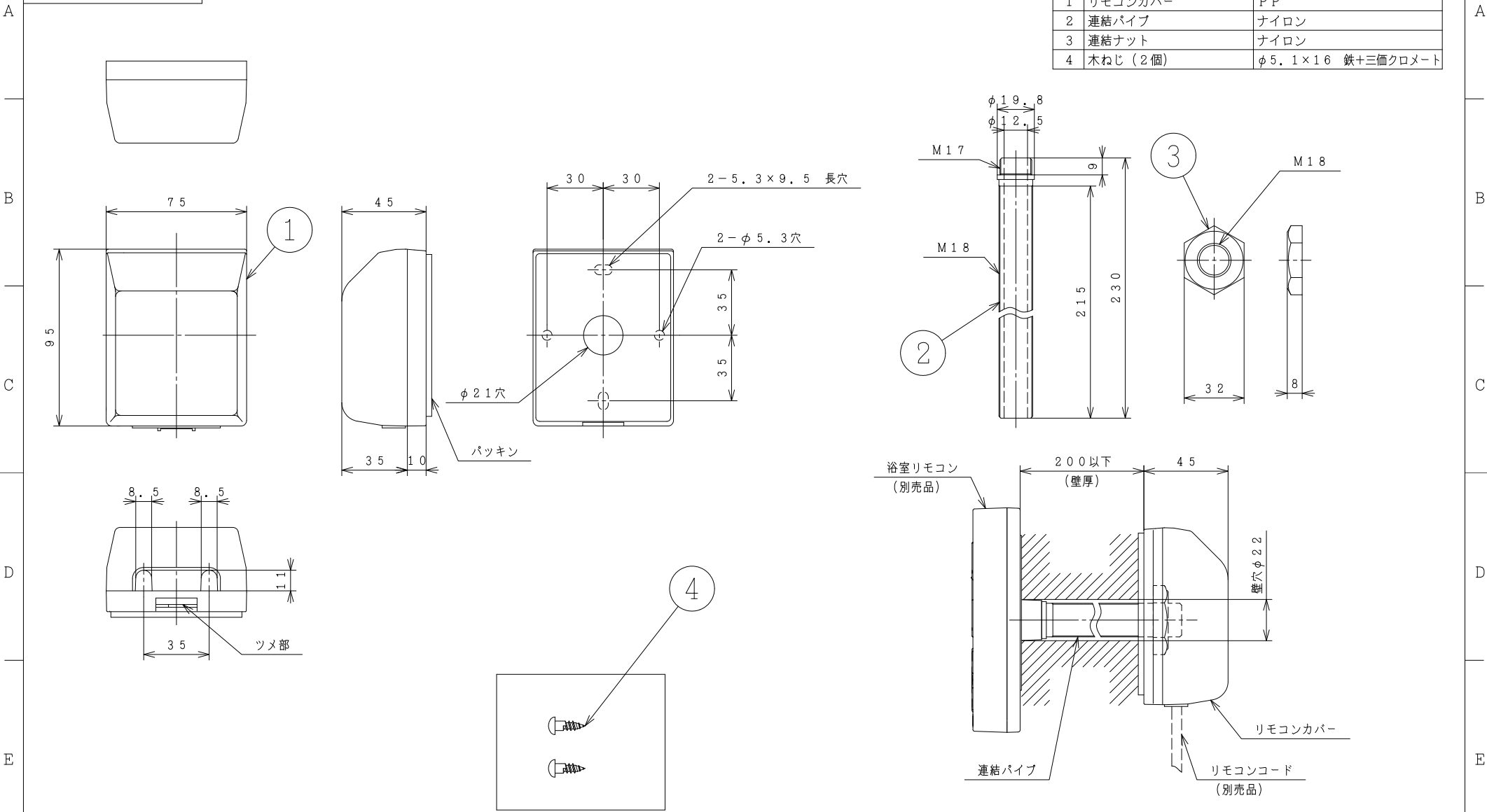
リモコンカバー、連結パイプ取付図
