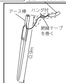
アース線の太さ 導線1.6φ又は2mm 2 以上
