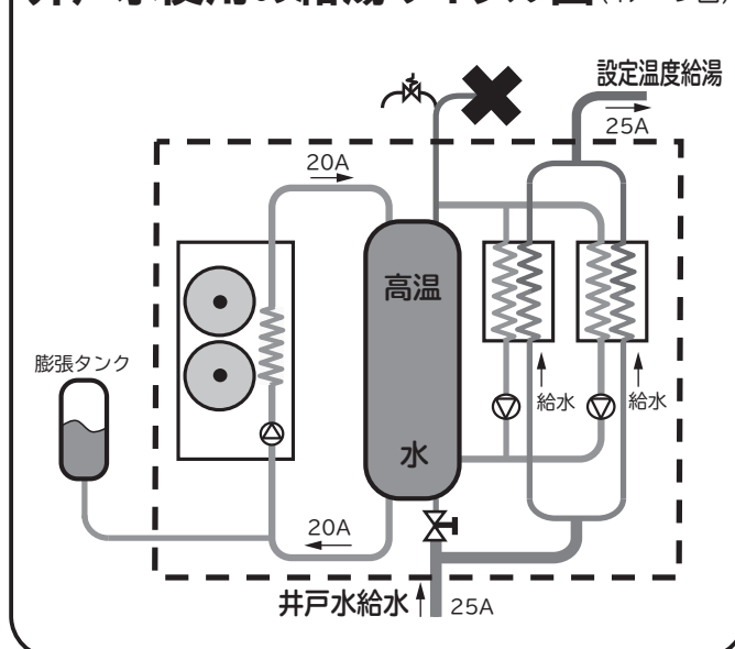
井戸水使用の給湯サイクル図（イメージ図）
