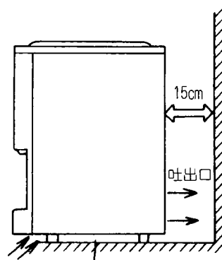
空気吸込口 底面のすき間
