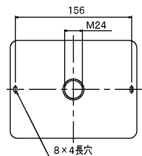
取付寸法図
