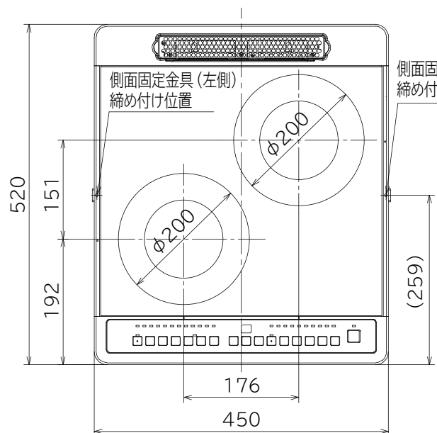
上面図
