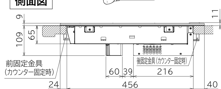
側面図
