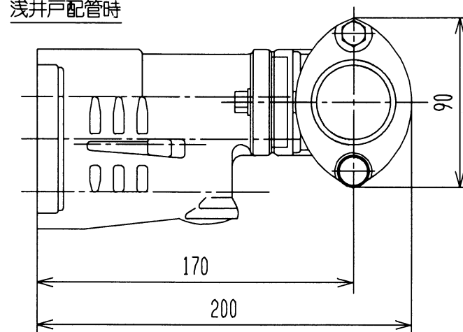
浅井戸配管時
