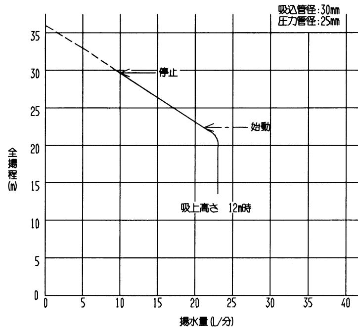
深井戸 シングルジェット (J25-18SH1) 使用時
