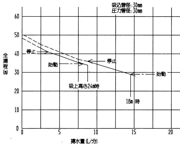
深井戸 専用ジェット (J25-24J) 使用時
