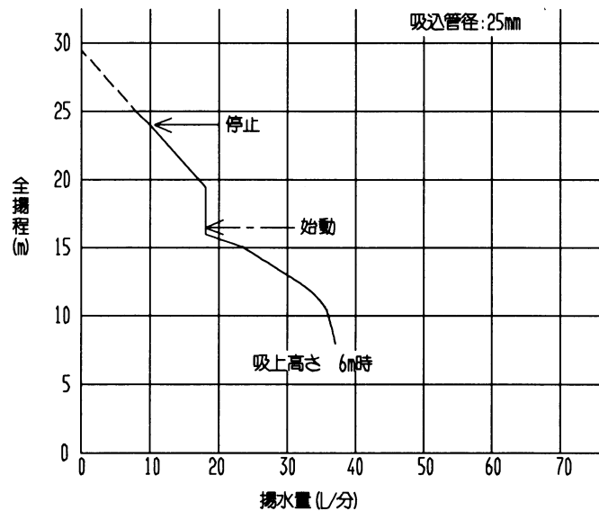
深井戸 専用ジェット (J25-24J) 使用時
