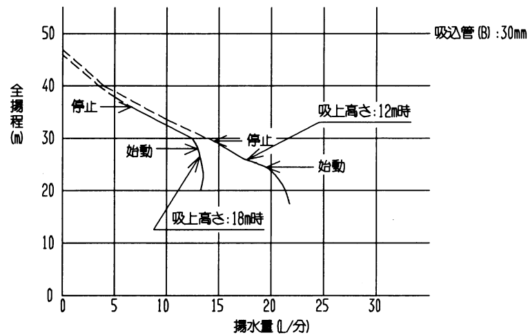
深井戸 シングルジェット (J25-18SH1) 使用時
