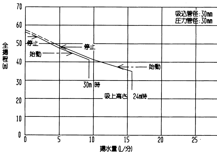
深井戸
