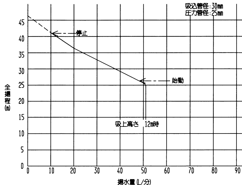
深井戸 専用ジェット (J75-35J) 使用時
