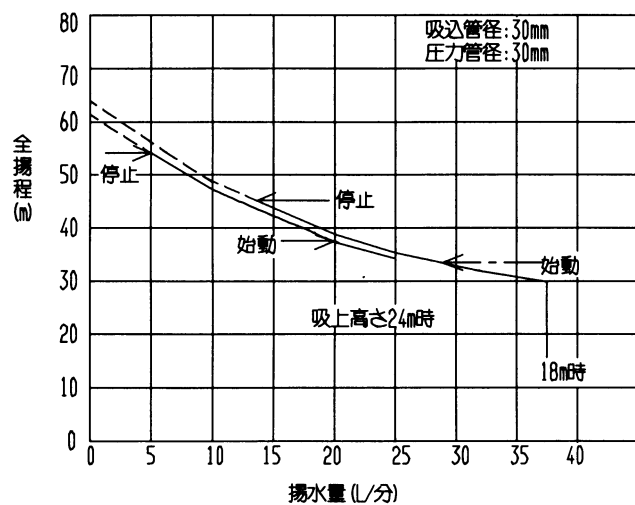
深井戸 専用ジェット (J75-24J) 使用時
