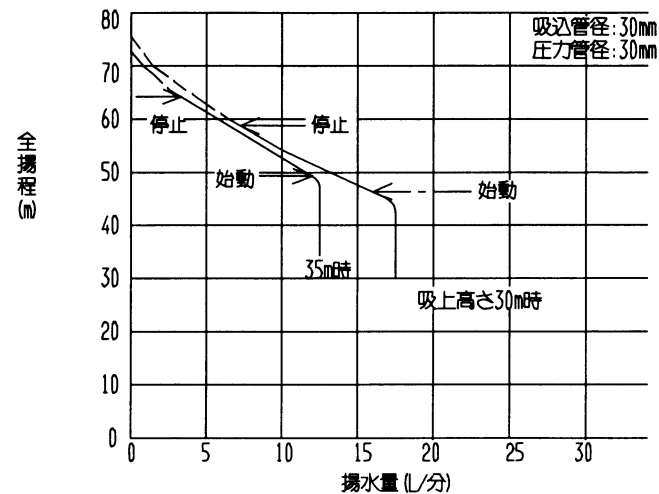
深井戸 専用ジェット (J75-35J) 使用時
