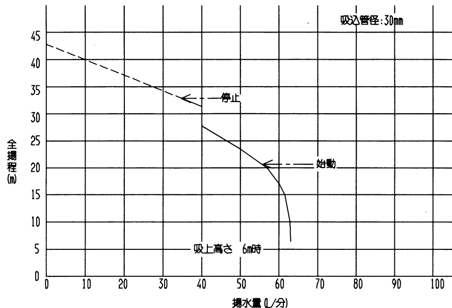
浅井戸配管 標準ジェット (J75-6J) 使用時
