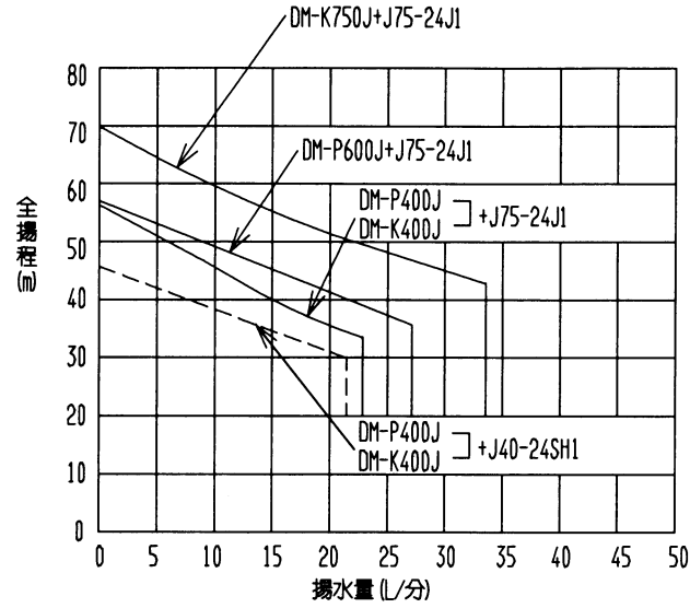
吸上げ高さ35m時の場合 (DM-P600J, DM-K750J)
