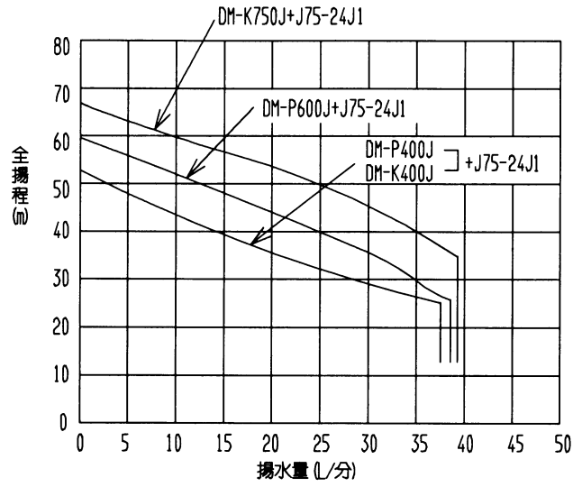
吸上げ高さ30m時の場合
