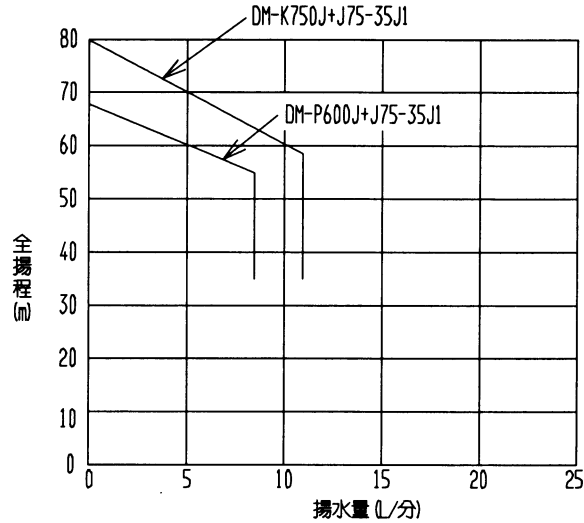
吸上げ高さ35m時の場合 (DM-P600J, DM-K750J)
