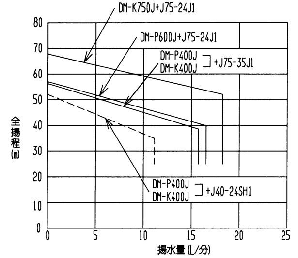
吸上げ高さ24m時の場合
