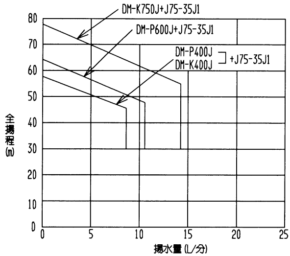
吸上げ高さ30m時の場合
