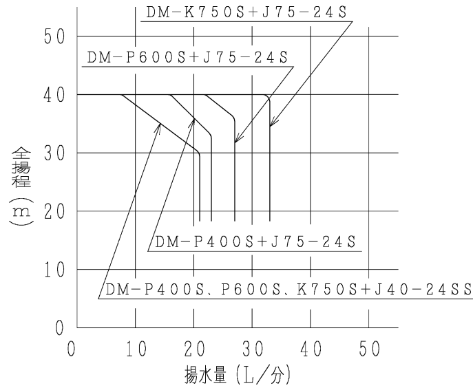
吸上高さ35m時の場合 (DM-P600S, K750S)
