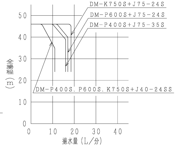
吸上高さ24m時の場合
