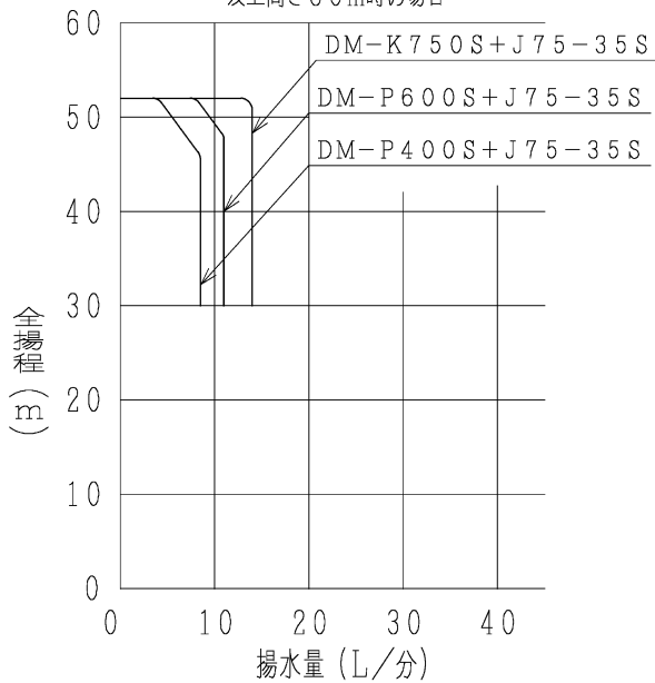
吸上高さ30m時の場合
