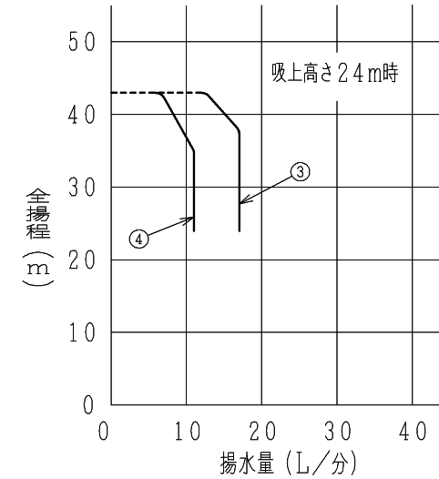
③深井戸専用ジェット (J75-24V) 使用時 ④深井戸用シングルジェット (J40-24SV) 使用時
