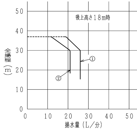
①深井戸専用ジェット (J75-24V) 使用時 ②深井戸用シングルジェット (J40-24SV) 使用時
