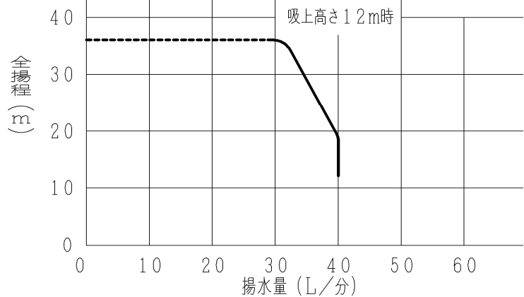
深井戸配管 標準ジェット (J40-6W) 使用時 吸込管径: 30mm 圧力管径: 25mm
