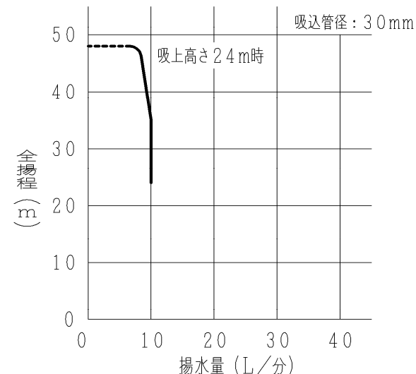
深井戸 シングルジェット (J40-24SW) 使用時
