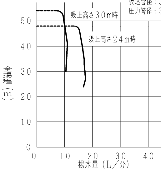
深井戸配管 標準ジェット (J40-6W) 使用時 吸込管径: 30mm 圧力管径: 25mm
