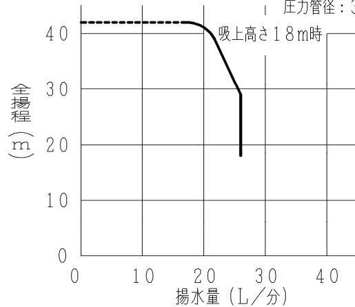
深井戸 専用ジェット (J75-35W) 使用時 吸込管径: 30mm 圧力管径: 30mm
