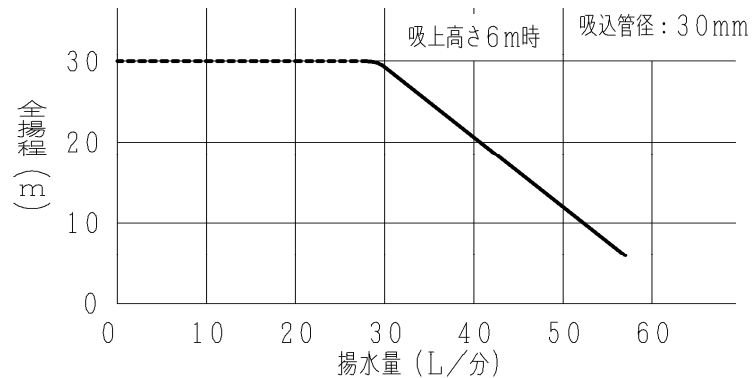
浅井戸配管 標準ジェット (J40-6W) 使用時
