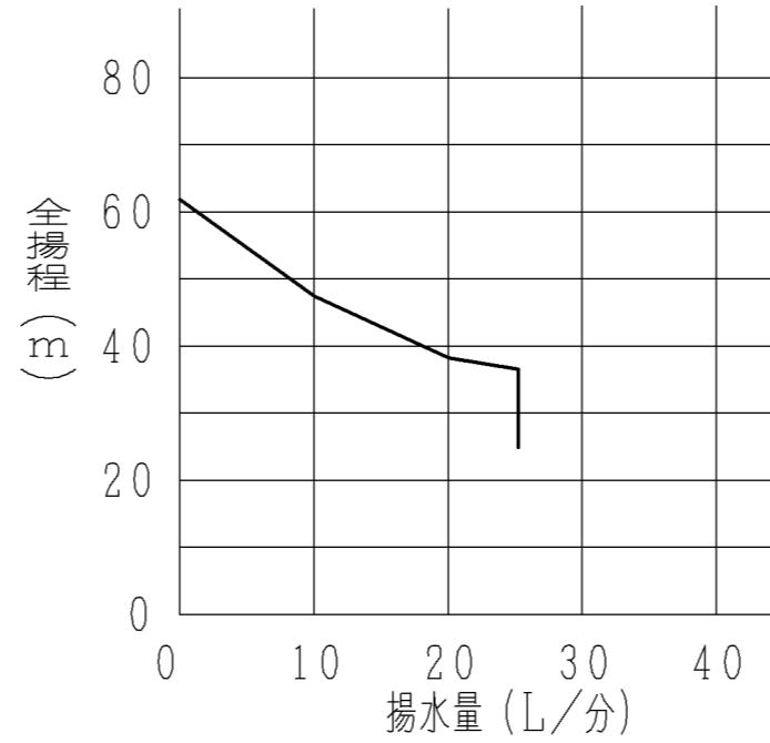
【深井戸ジェットJ75-24X組合わせ時】 吸上高さ24m
