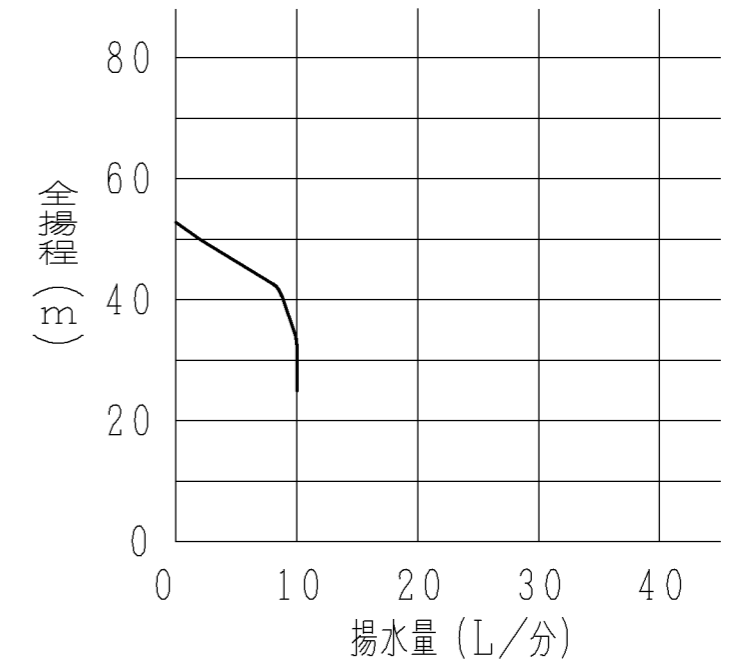
【深井戸用特殊ジェットJ40-24SX組合わせ時】 吸上高さ24m
