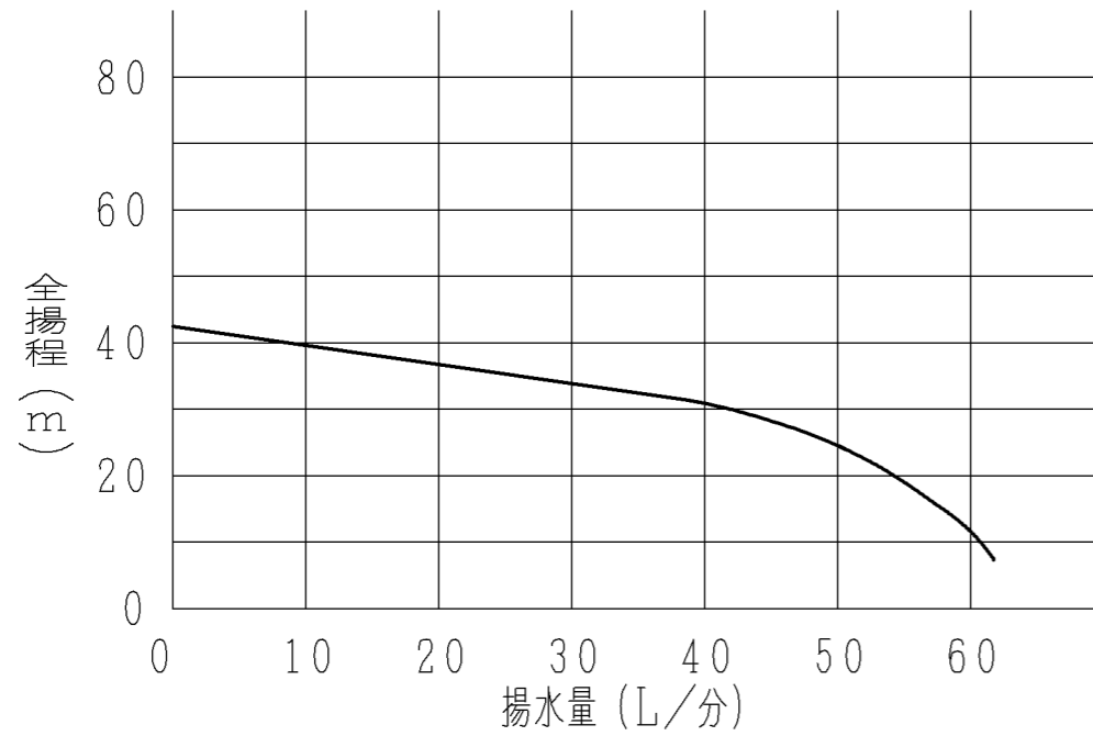
【標準ジェットJ75-7Y組合わせ時】 吸上高さ6m
