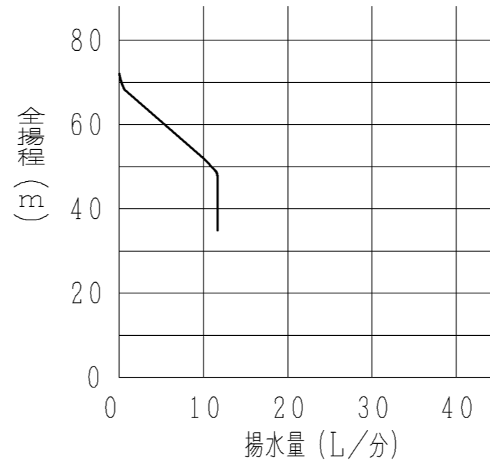
【深井戸ジェットJ75-35X組合わせ時】 吸上高さ35m
