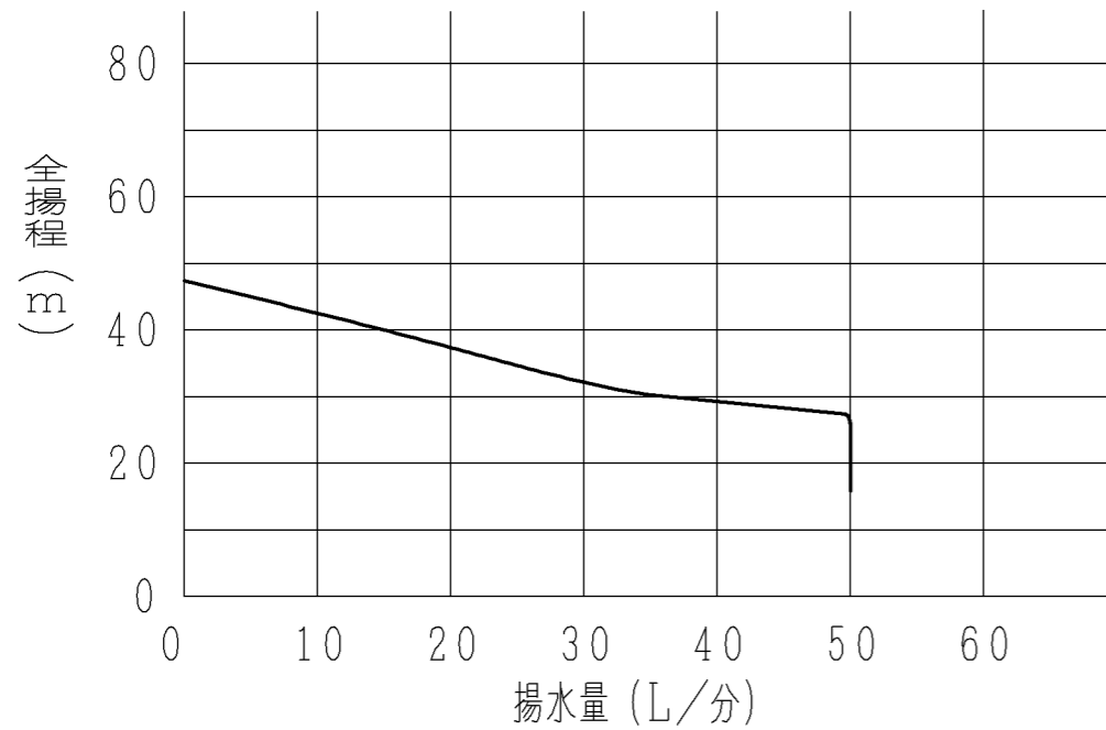
【標準ジェットJ75-7Y組合わせ時】 吸上高さ12m
