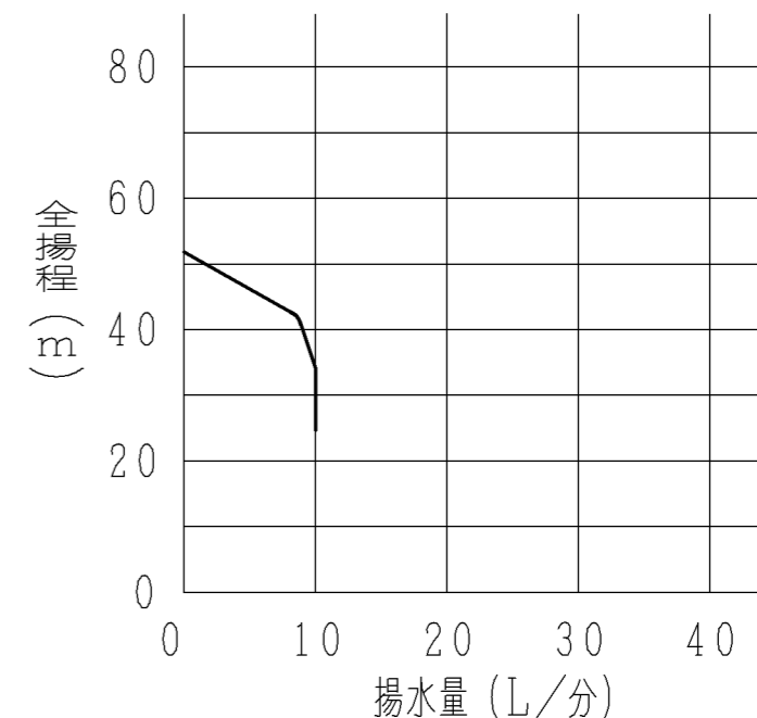
【深井戸用特殊ジェットJ40-24SX組合わせ時】 吸上高さ24m
