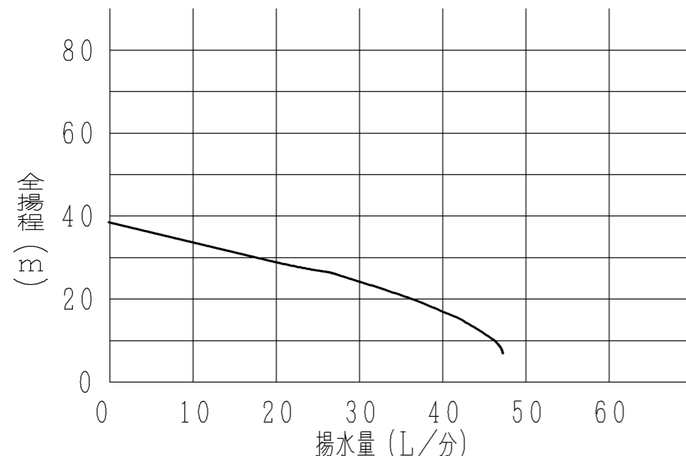
【標準ジェットJ40-7Y組合わせ時】 吸上高さ12m
