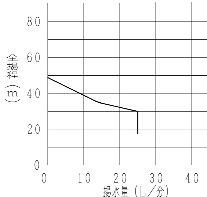
【深井戸ジェットJ75-24X組合わせ時】 吸上高さ18m
