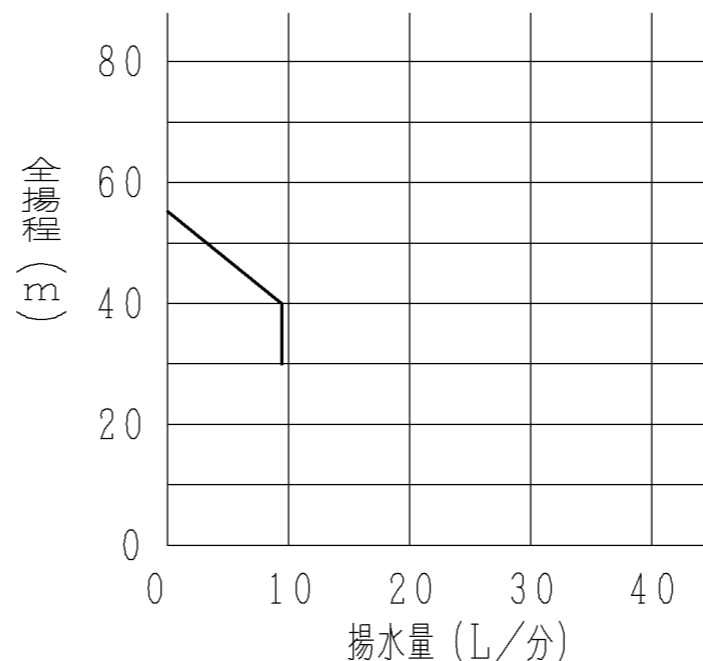
【深井戸ジェットJ75-35X組合わせ時】 吸上高さ30m
