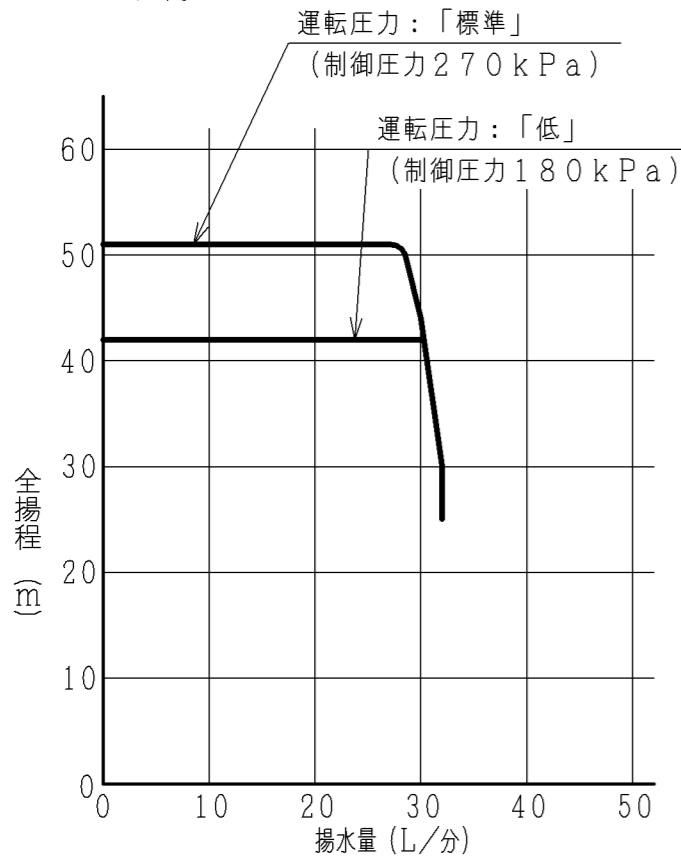
【深井戸ジェットJ75-24X組合わせ時】 吸上高さ24m
