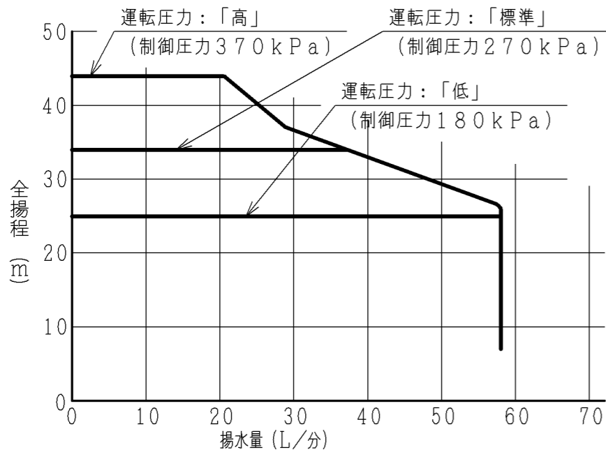
【深井戸ジェットJ75-24X組合わせ時】 吸上高さ24m
