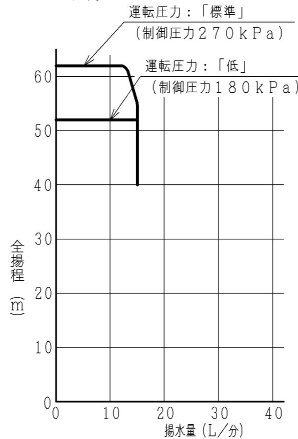
【深井戸ジェットJ75-35X組合わせ時】 吸上高さ35m
