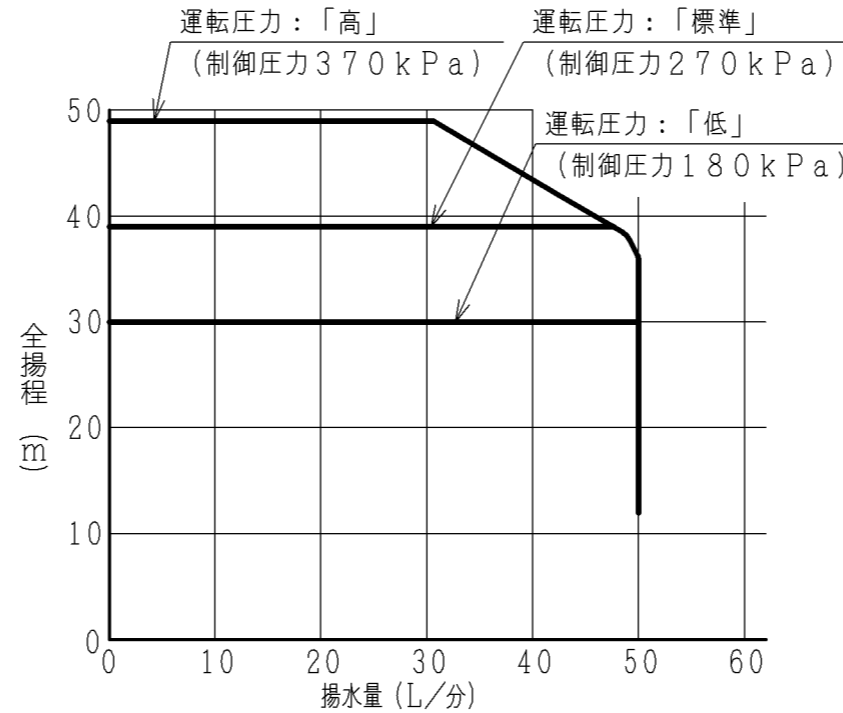
【深井戸ジェットJ75-35X組合わせ時】 吸上高さ35m
