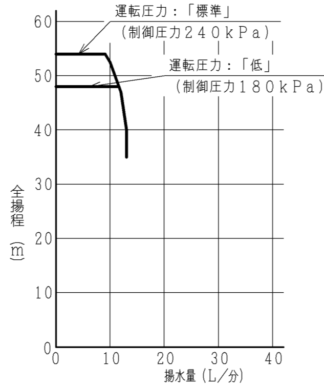
【深井戸ジェットJ75-35X組合わせ時】 吸上高さ30m
