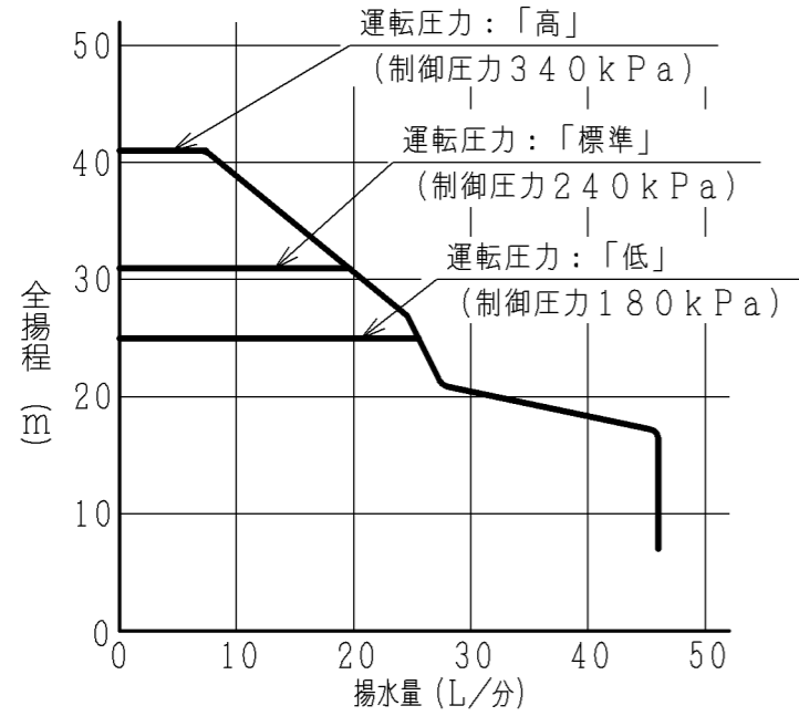
△【標準ジェットJ40-7Y組合わせ時】 吸上高さ7m
