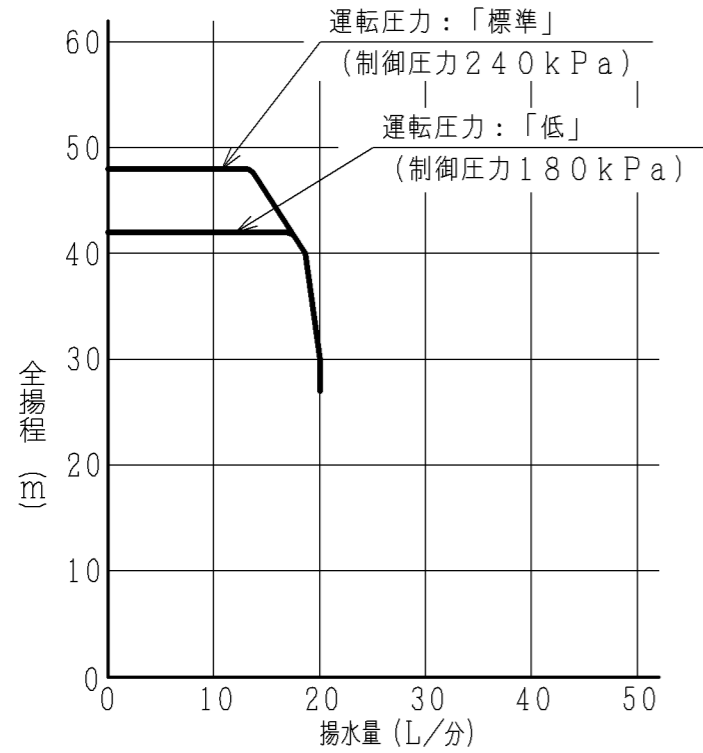
【深井戸ジェットJ75-24X組合わせ時】 吸上高さ24m
