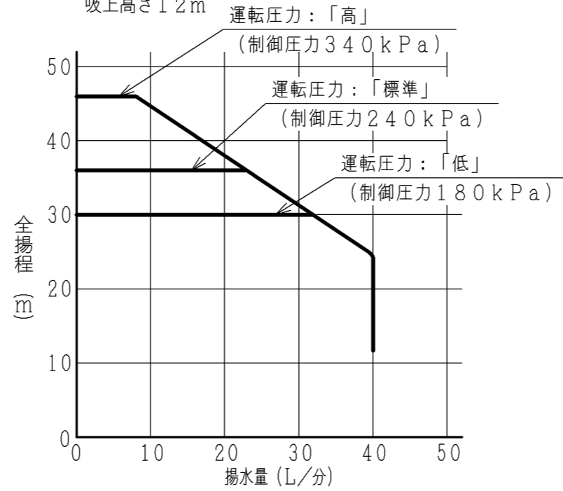
△【標準ジェットJ40-7Y組合わせ時】 吸上高さ12m
