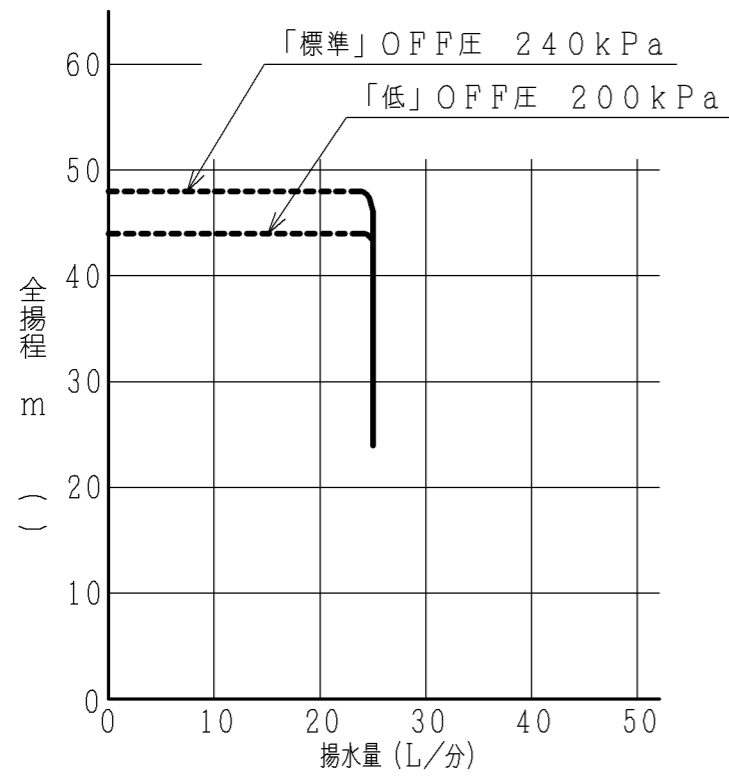
【浅井戸ジェットJ75-24X組合わせ時】 吸上高さ24m
