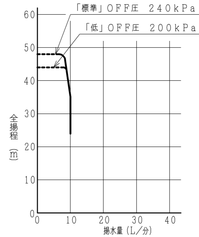
浅深両用自動ポンプ(750W)揚水性能
