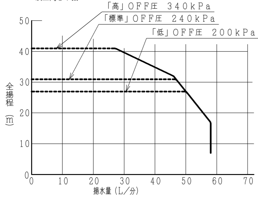
【浅井戸ジェットJ75-24X組合わせ時】 吸上高さ24m
