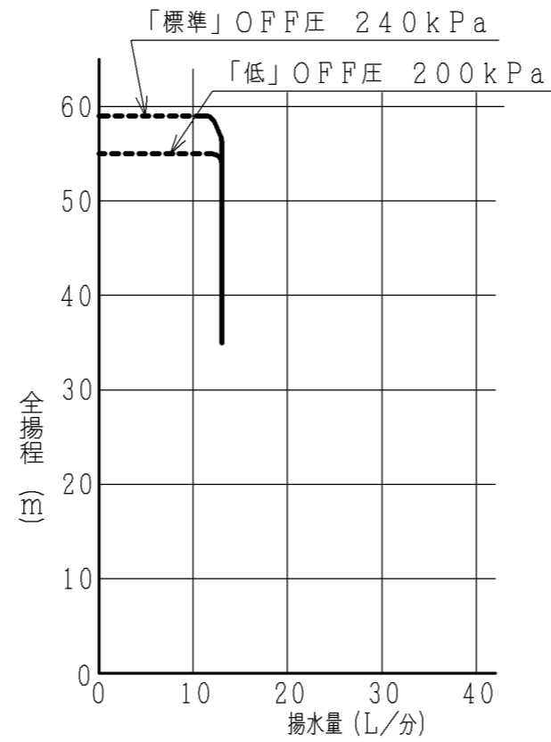
【浅井戸ジェットJ75-35X組合わせ時】 吸上高さ35m
