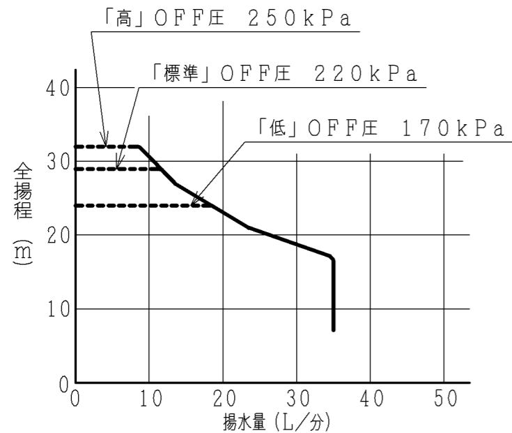
【浅井戸ジェットJ25-12Y組合せ時】 吸上高さ7m時
