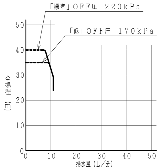
【深井戸用特殊ジェットJ25-18SX組合せ時】 吸上高さ18m時
