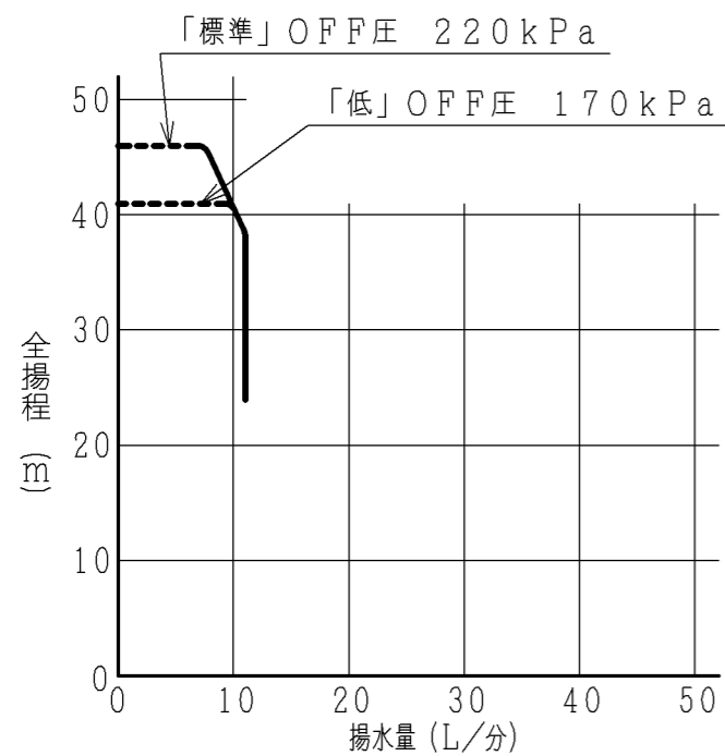
【浅井戸ジェットJ25-24X組合せ時】 吸上高さ24m時
