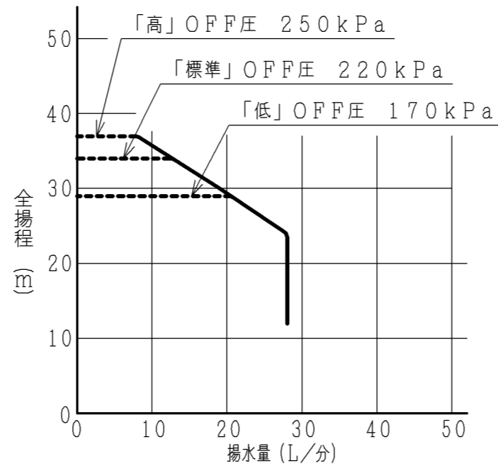
【深井戸ジェットJ25-12Y組合せ時】 吸上高さ12m時
