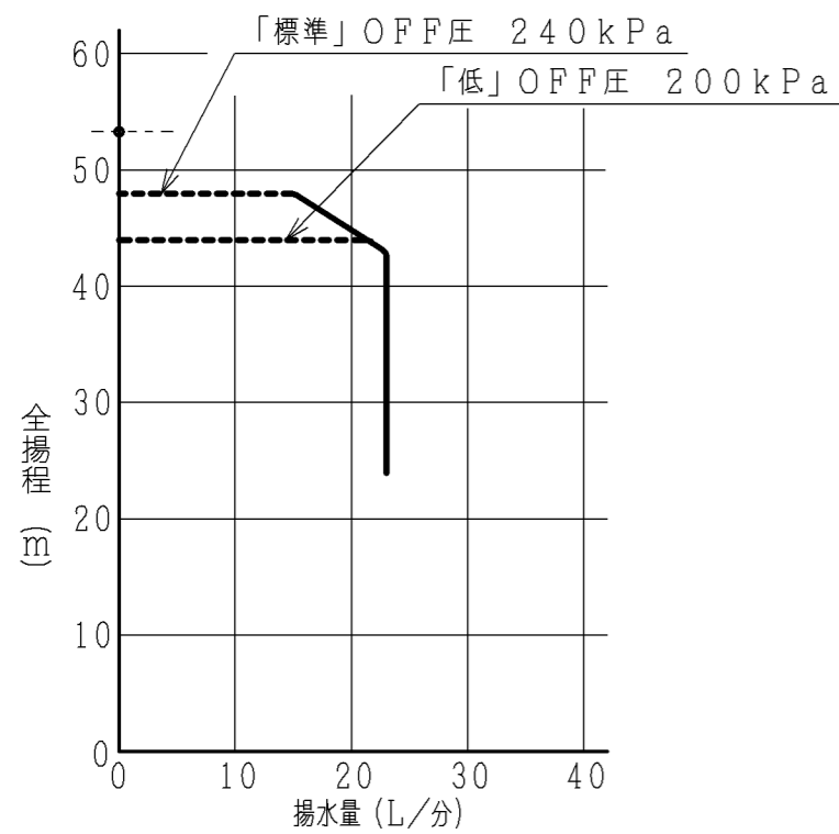
【浅井戸ジェットJ75-24X組合わせ時】
