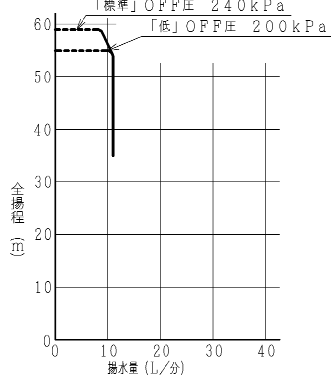
【浅井戸ジェットJ75-35X組合わせ時】
