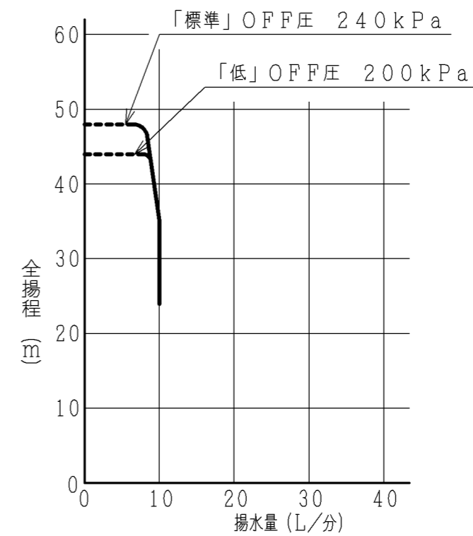
【深井戸用特殊ジェットJ40-24SX組合わせ時】
