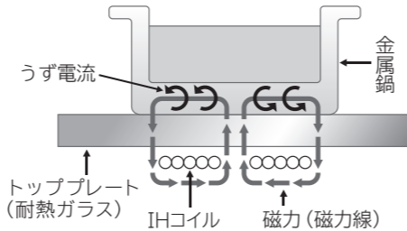
IH加熱の原理(イメージ図)
