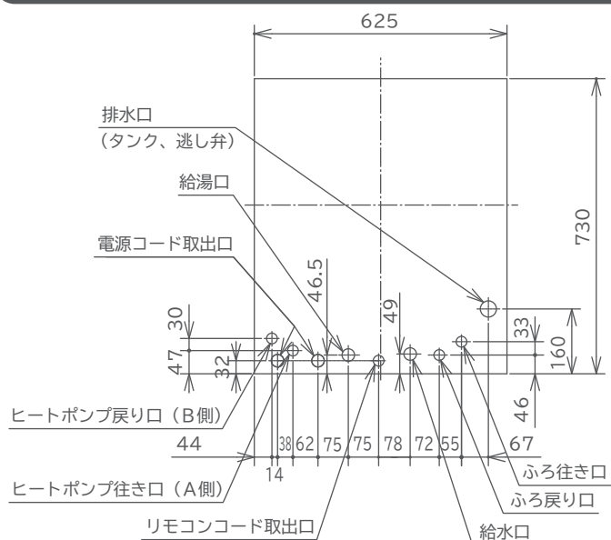
配管取り出し位置図
