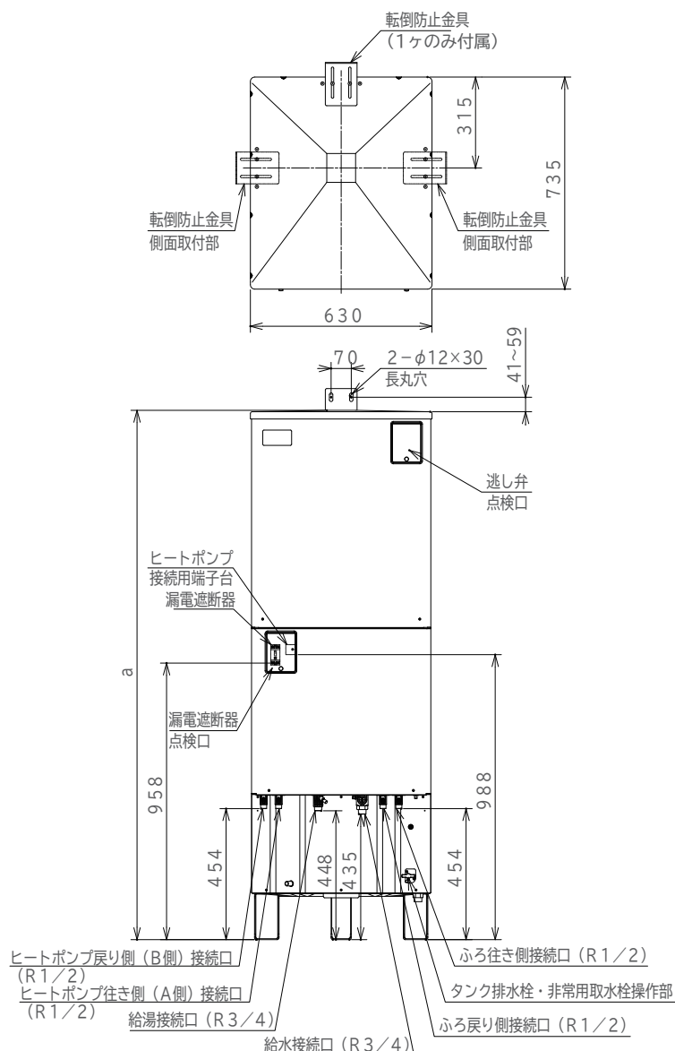
配管取り出し位置図
