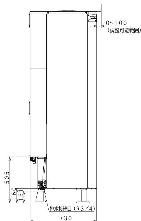
貯湯ユニット脚部寸法
