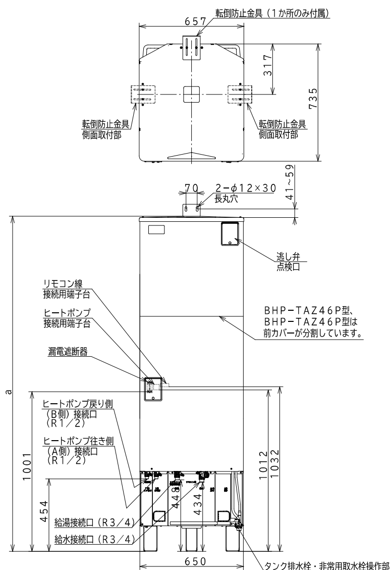
配管取り出し位置図
