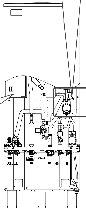
漏電遮断器
