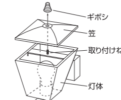
22 ギボシねじ式
