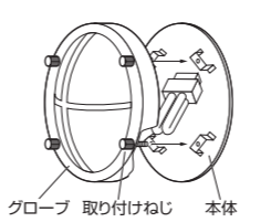
25 正面ねじ式
