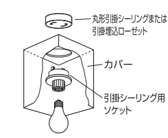
28 引掛け式
