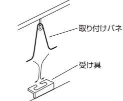
7 Vばね式
