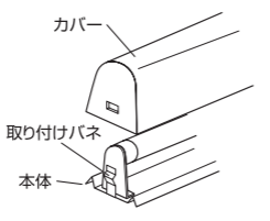
15 端面バネ止め式
