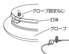
3 上ねじ式
