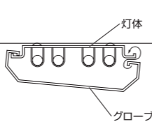
8 落としこみ式
