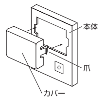
13 ツメ止め式
