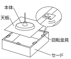
29 回転金具式
