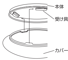
5 回転式
