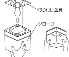
17 はめこみ回転式
