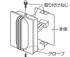
23 上下ねじ式
