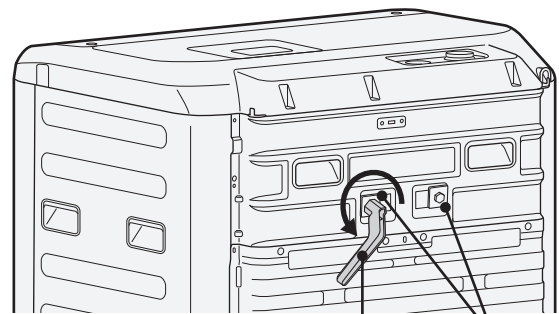
輸送用ボルト取り外しスパナ 輸送用ボルト
