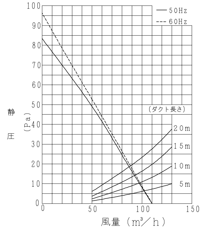
■ 風量-静圧特性
