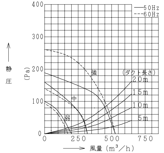
■ 風量-静圧特性
