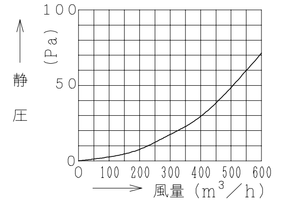
■ 圧力損失特性
