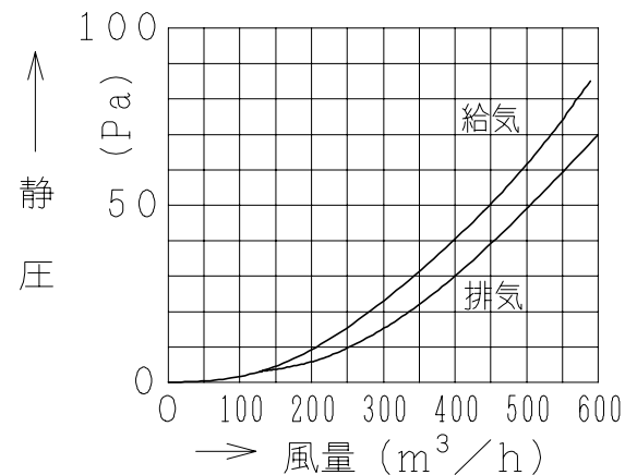
■ 圧力損失特性
