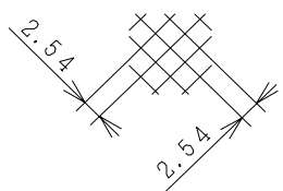
■ 防虫網詳細
