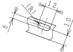
P (横幕板→本体固定用長穴)
