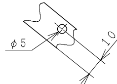
Q (横幕板→本体固定用穴)
