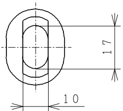
防振ゴム拡大図
