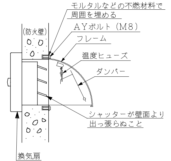
取り付け例
