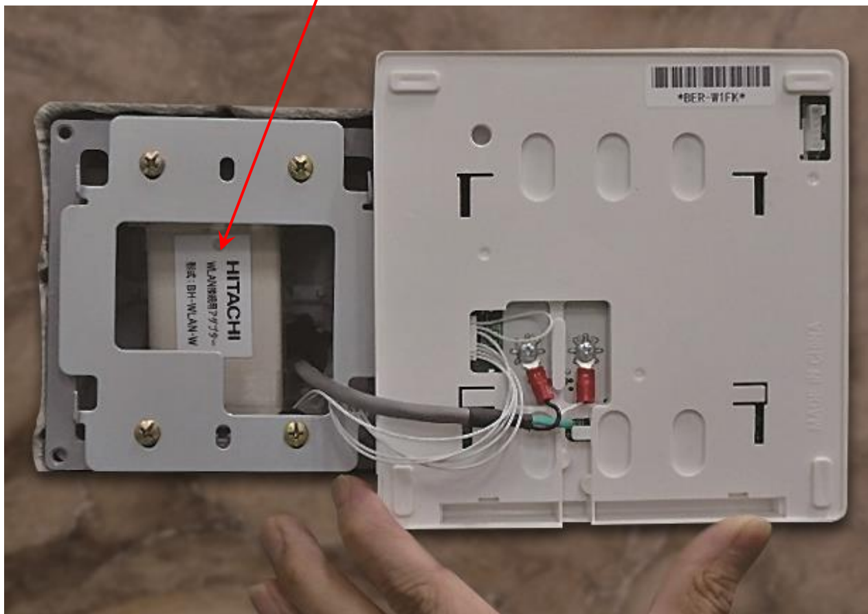
無線LANアダプター BH-WLAN-W の設置写真撮影例
