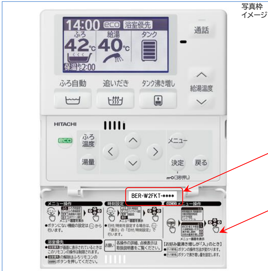
無線LANアダプター付属リモコン BER-W2FH-Tの 台所リモコン「BER-W2FKT」の設置写真撮影例
