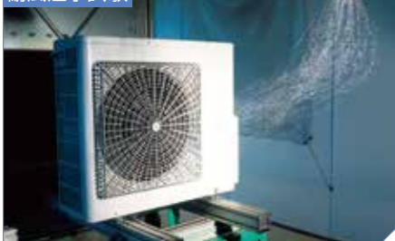
耐風注水試験
