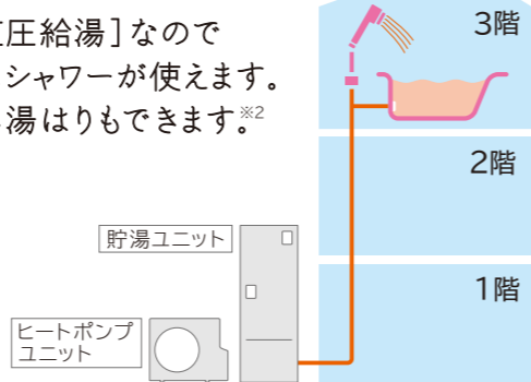
※2 お風呂の湯はりはタンクから給湯します。3階での湯はりの場合は、3階浴そう用水流スイッチ(別売)が必要です。
