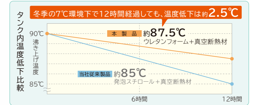
※当社調べ。タンク湯温を90°Cに沸き上げ運転後、7°C環境下に12時間放置したあとのタンク湯温を当社従来製品BHP-FV37ND(2013年発売)と比較。
