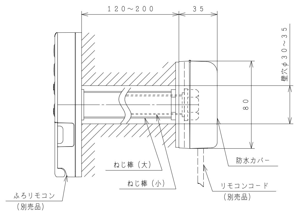
防水カバー、ねじ棒 (大) (小) 取付図
