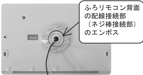
ふろリモコン背面部
