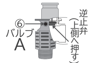
逆止弁位置(給水継手左視図)
