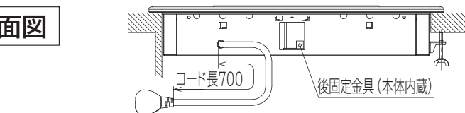
側面図
