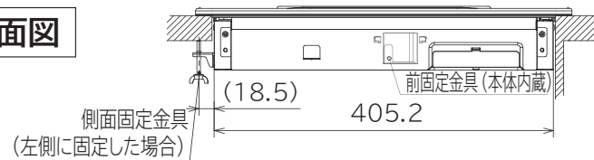
後面図
