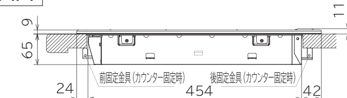
側面図
