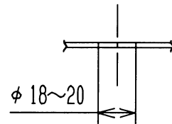
満水警報器取付穴形状
