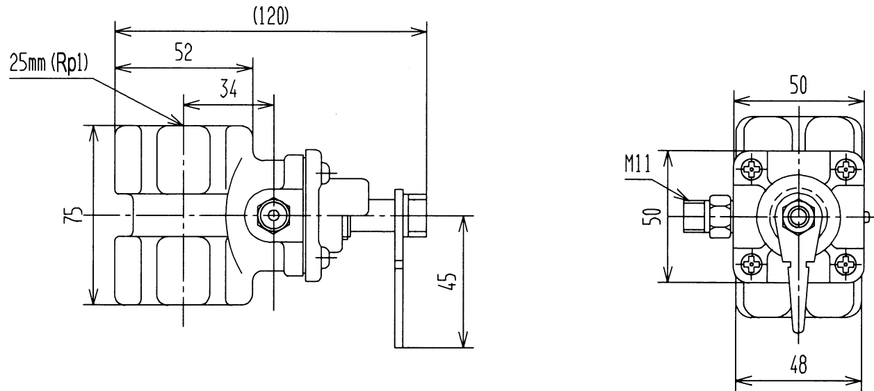
(降水器本体)
