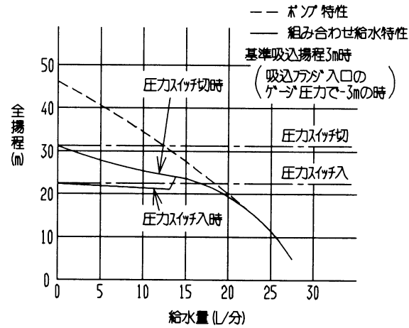
WT-PL200J・PUS-320LJとの組み合わせ揚水性能曲線
