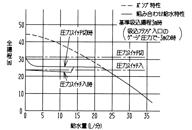
WT-PL300J・PUS-330LJとの組み合わせ揚水性能曲線
