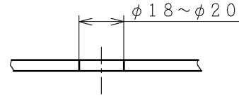
満水警報器取付穴形状
