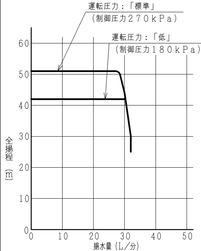
【深井戸ジェットJ75-24Y組合わせ時】 吸上高さ24m
