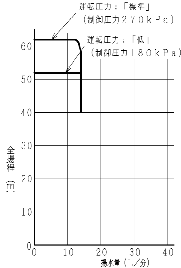
【深井戸ジェットJ75-35Y組合わせ時】 吸上高さ35m
