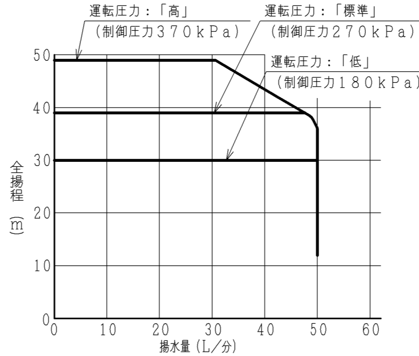
【深井戸ジェットJ75-35Y組合わせ時】 吸上高さ35m
