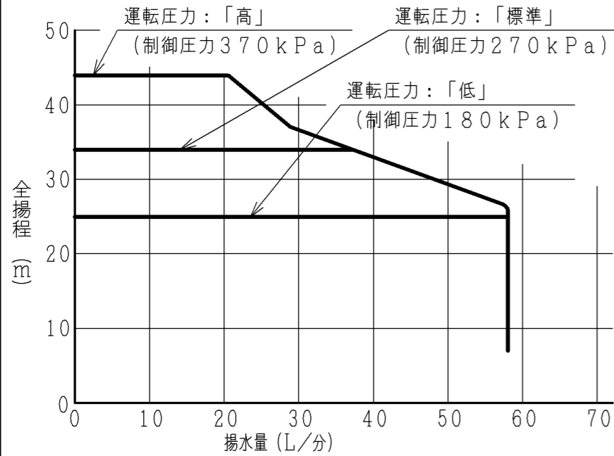
【深井戸ジェットJ75-24Y組合わせ時】 吸上高さ24m
