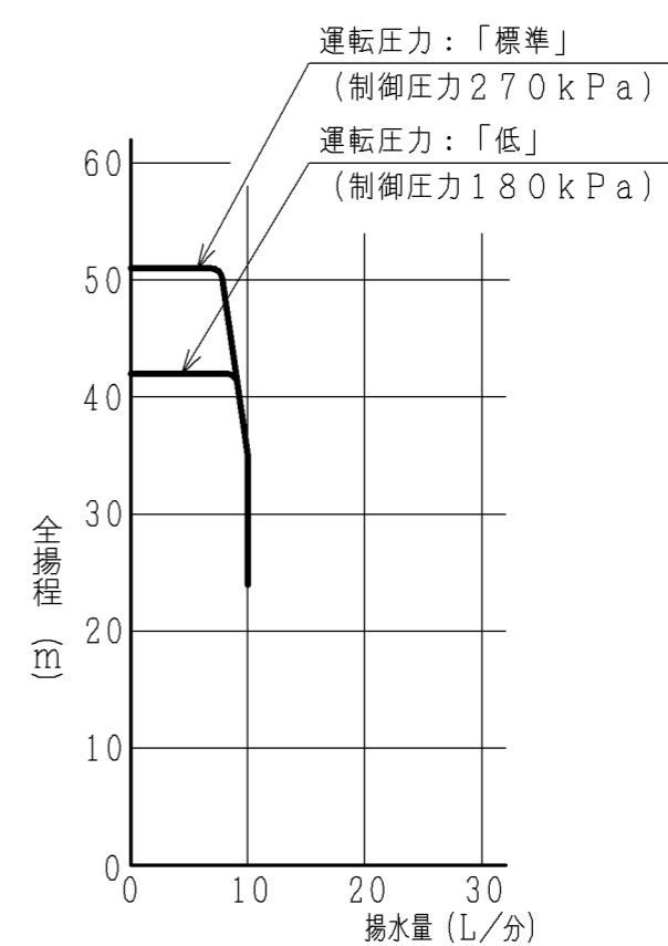
【特殊ジェットJ40-24SX組合わせ時】 吸上高さ24m
