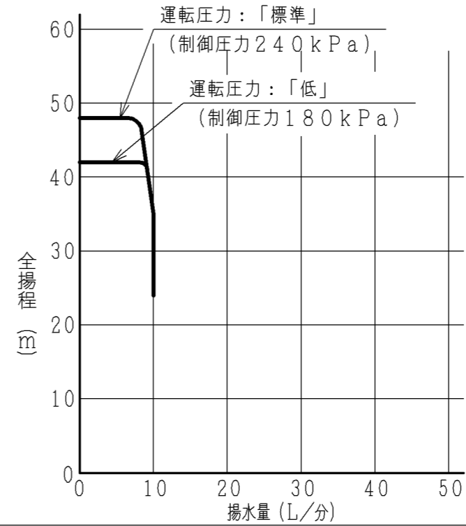
浅深両用自動ポンプ (ミニタンク式) CM-P400Y 揚水性能
