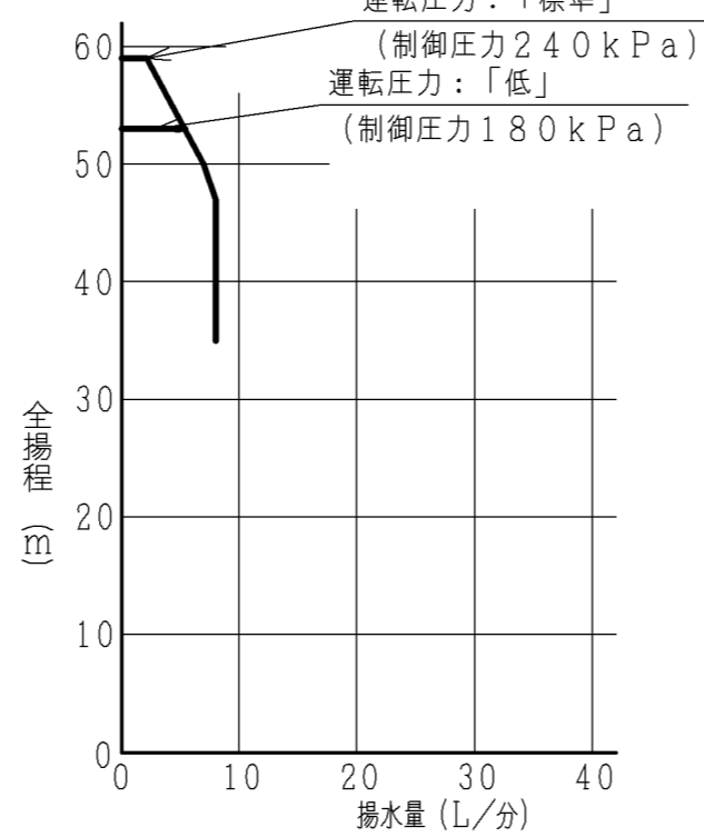
【深井戸ジェットJ75-35Y組合わせ時】 吸上高さ35m
