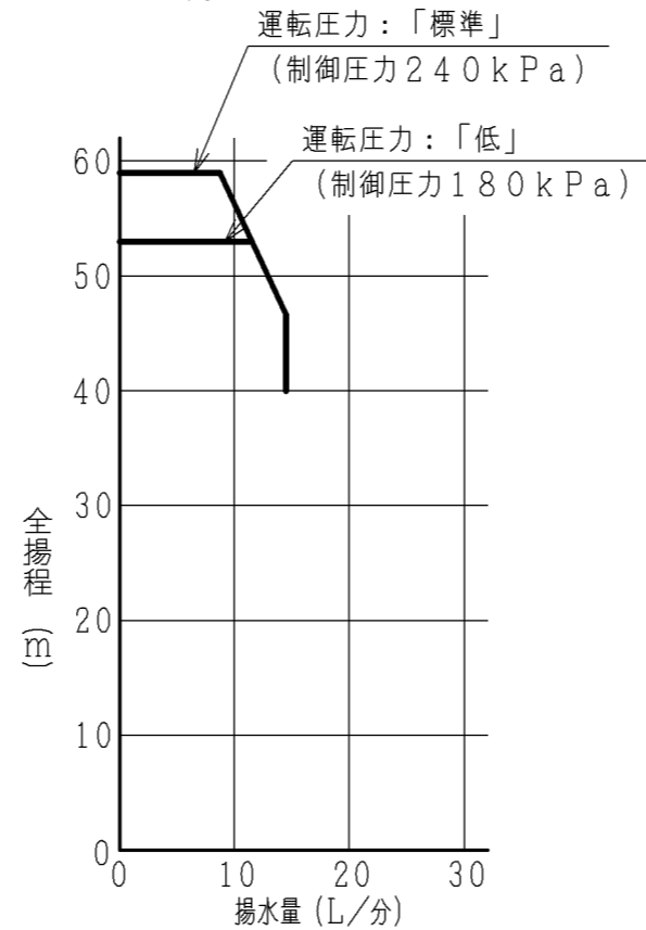
【深井戸ジェットJ75-35Y組合わせ時】 吸上高さ35m
