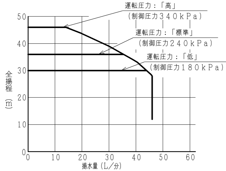
【深井戸ジェットJ75-35Y組合わせ時】 吸上高さ35m
