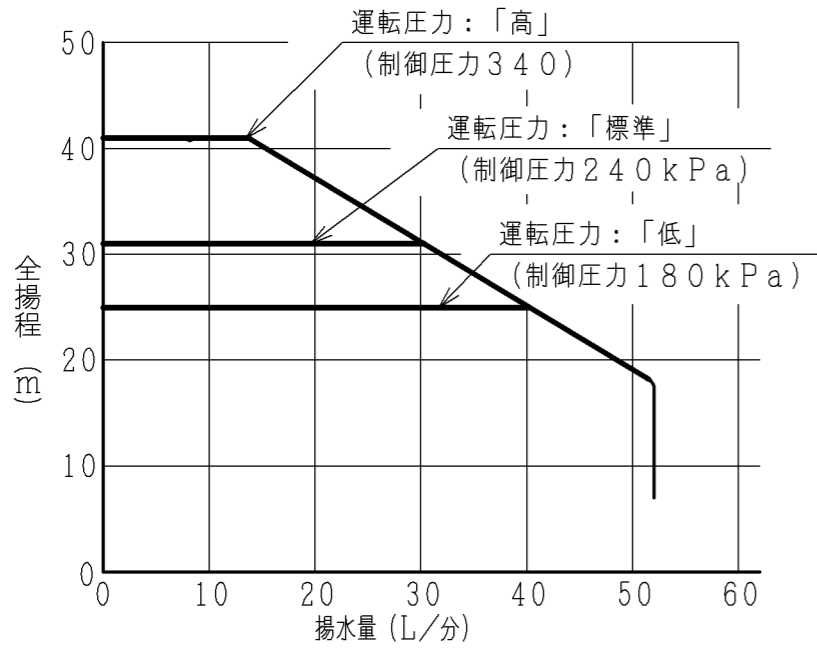
【深井戸ジェットJ75-24Y組合わせ時】 吸上高さ24m
