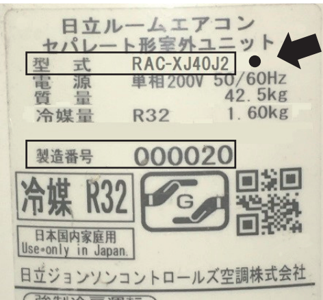
【本体仕様銘板】
